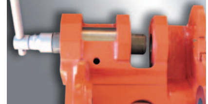
Verriegelungsbolzen mit 1 1/2 Umdrehungen öffnen
