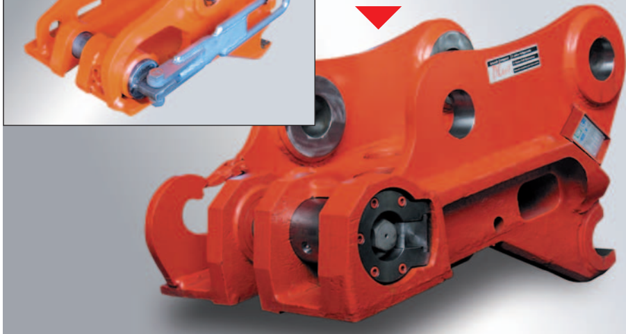
A-Lock mech Compact, Kl 3, 3 C Sechskantaufsatz, keine seitlich vorstehenden Elemente
