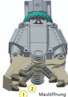
TOPCUT mit Dino-Gebiss
