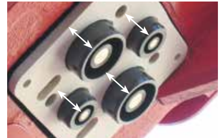
2-Schritt-Technik: Erst nach dem Verriegeln des Werkzeuges werden die Kupplungen ausgefahren und verbinden die Hydraulikkreise.
