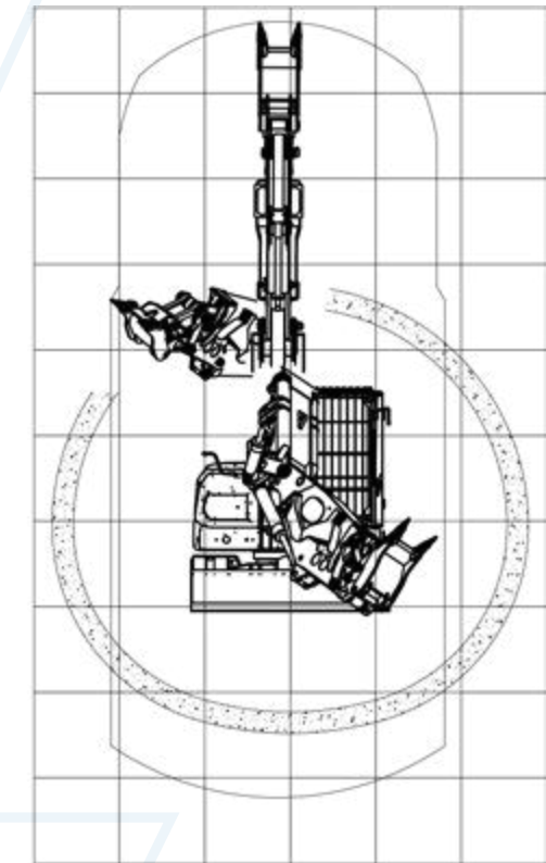
Fräseinsatz e-Badger
