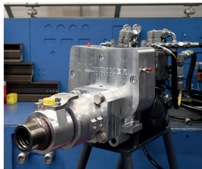
T23 Hammer ermöglicht drei verschiedenen Spülköpf-Varianten
