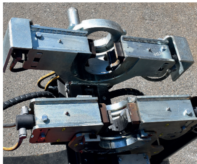
Klemm-Brechvorrichtung
