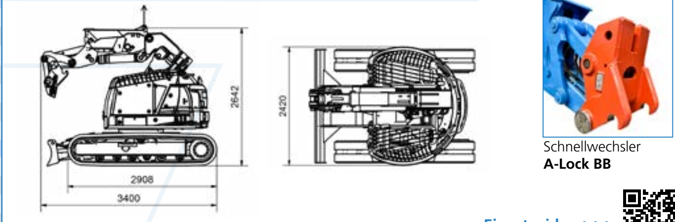
Abmessungen - Verladung mini-/e-Badger
