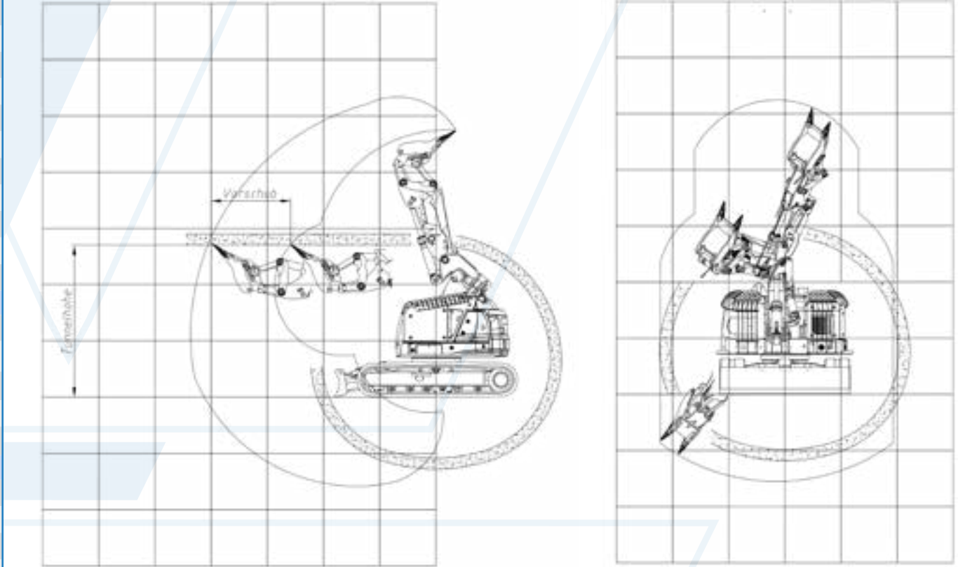
Abmessungen - Verladung mini-/e-Badger
