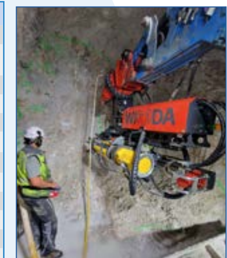
Einsatz im Tunnel WIDA AB C20 T-4
